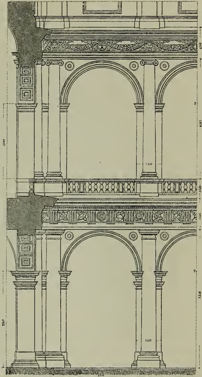
Abb. 211. Pal. Farnese zu Rom. Hofarkaden. (Nach Bühlmann.)
